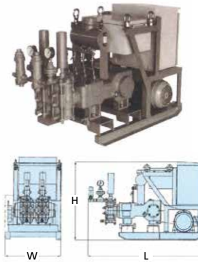
〈注入詳細イメージ〉
