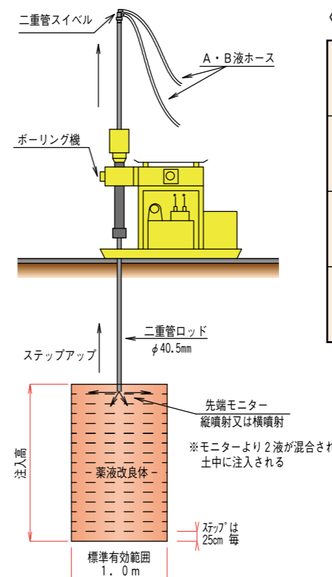
〈注入詳細イメージ〉
