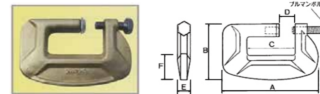
本体材質:S45C(鍛造品) 表面処理:電気亜鉛メッキ
