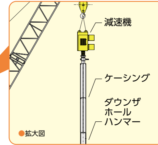
ノバルハンマー (セメントミルク注入可能)
