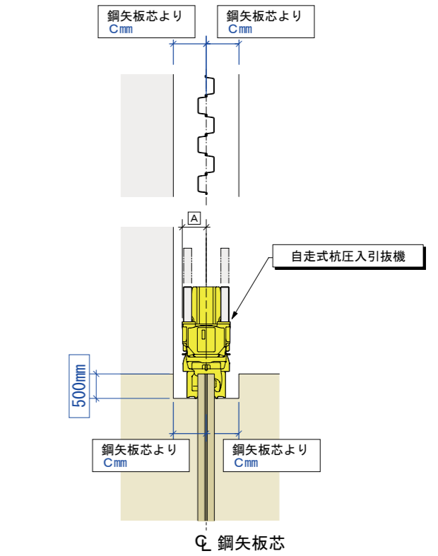
〈標準施工クリアランス ※補助工法・コーナー周りは異なります。〉
