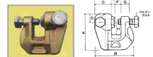
本体材質:S45C(鍛造品) 表面処理:電気亜鉛メッキ(JIS H8610 2種2級)
