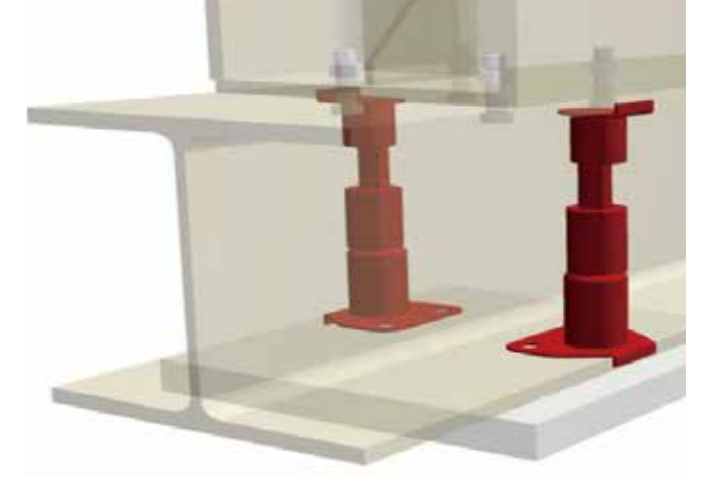
スティフナー補強の代替品として最適
