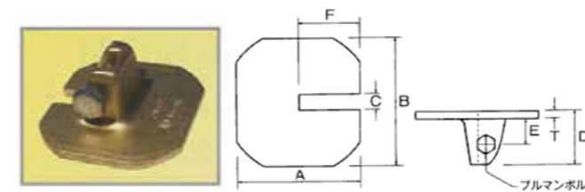
本体材質:S35C(鍛造品) 表面処理:電気亜鉛メッキ(JIS H8610 2種2級)
