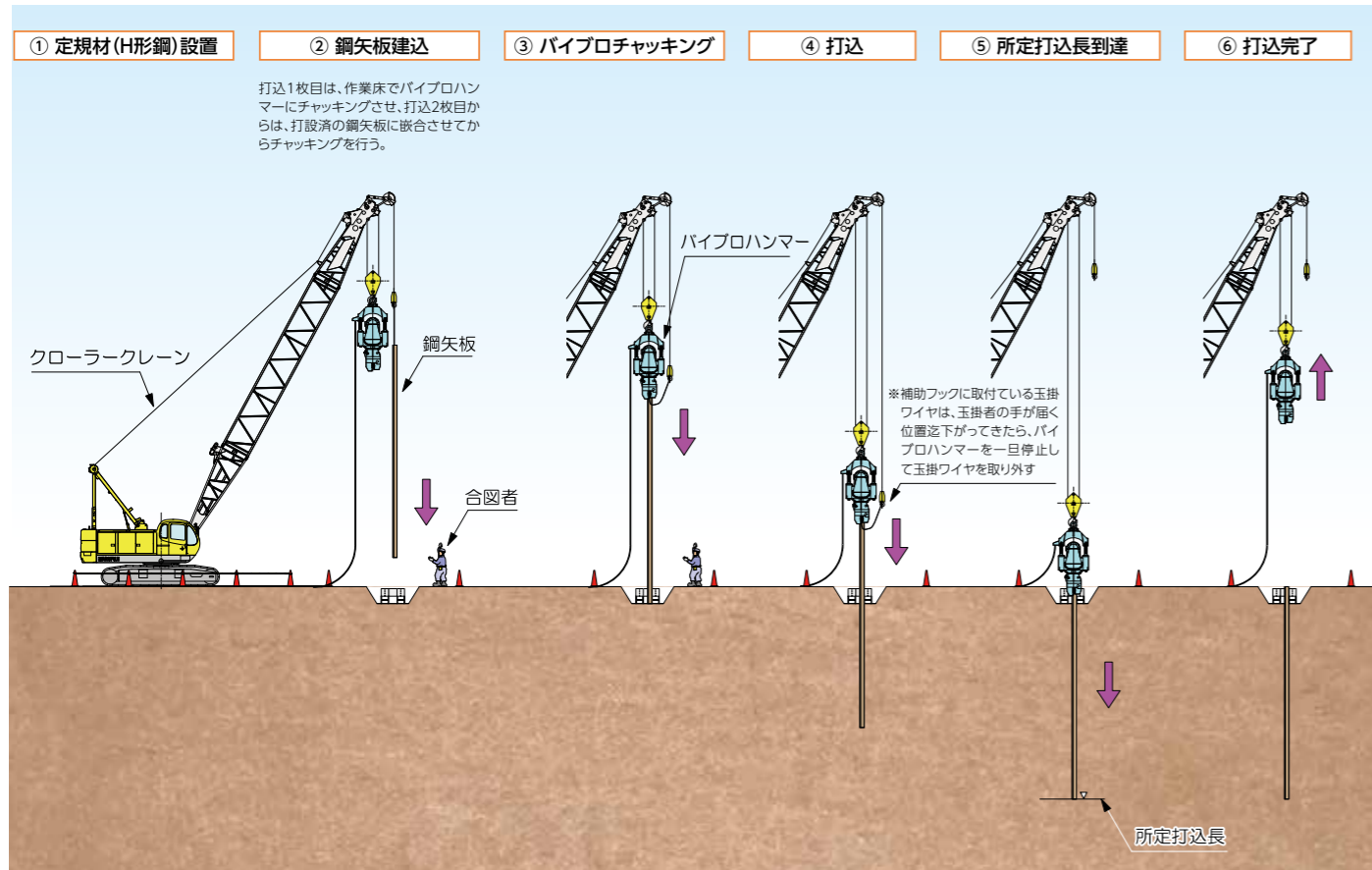
【施工フロー(クローラークレーン バイブロハンマー打込工)】
