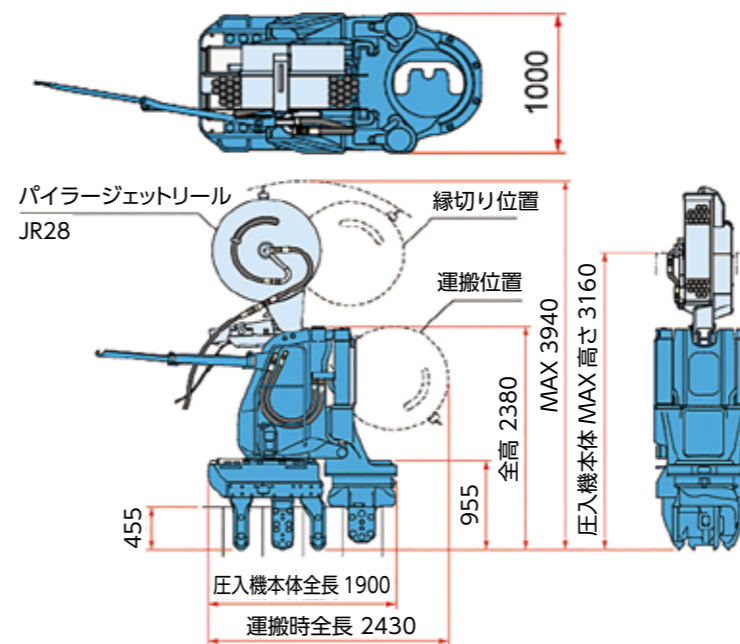
パワーユニット
