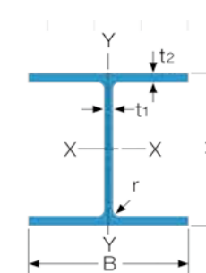
H形鋼(共通)
