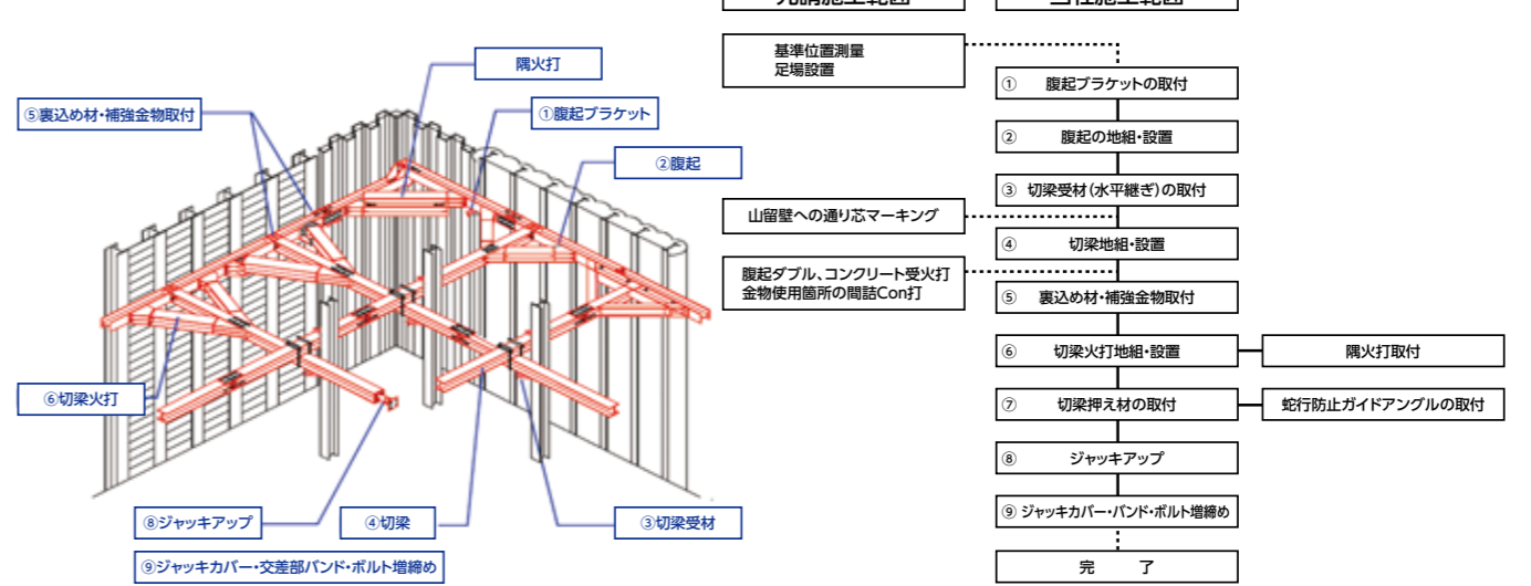
【施工フロー】
