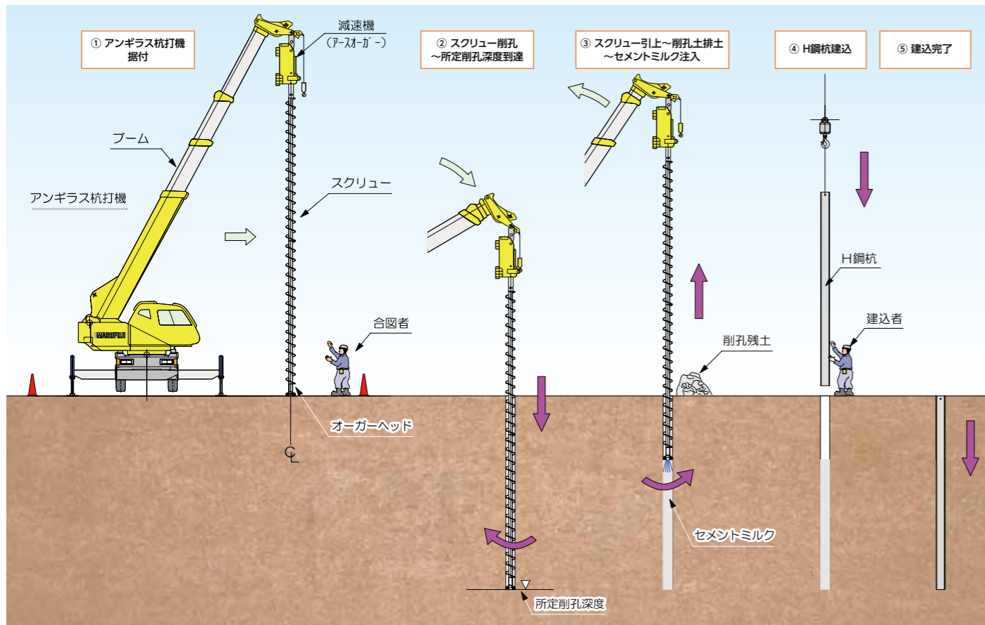
【施工フロー】
