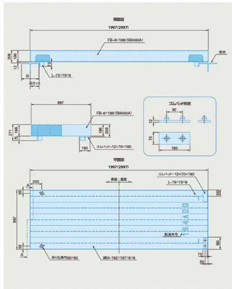
標準品構造図 1m×2m (1m×3m)
