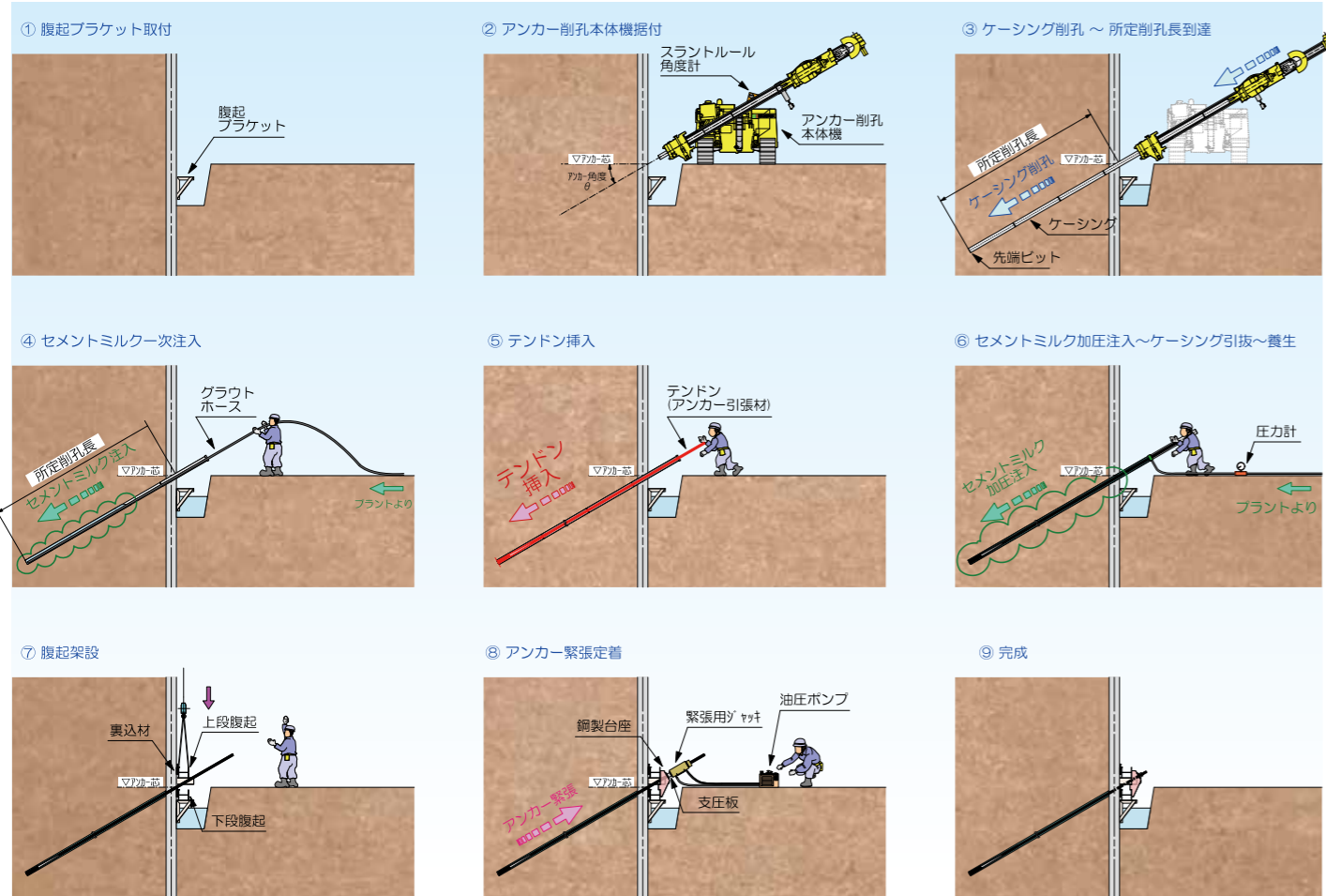
グラウンドアンカー打設状況
